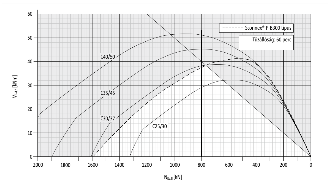
Ábra 43: Schöck Sconnex® P-B300 típus: interakciós ábra tűzesetre történő méretezéshez; R 60-as tűzállósági osztály
