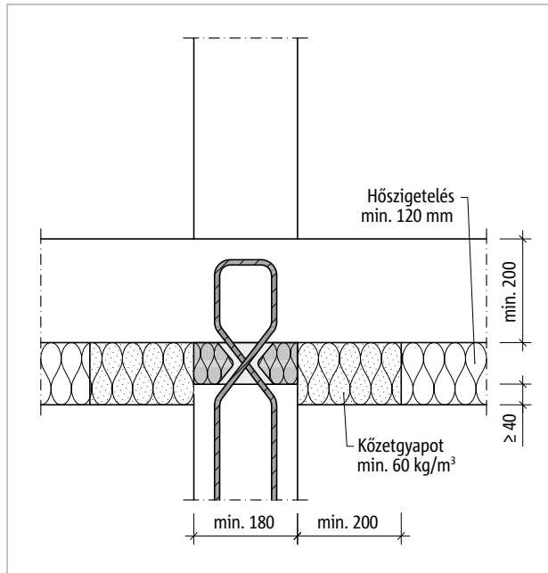
Ábra 139: Schöck Sconnex® W típus: kőzetgyapot szegélyszávvval a földem alsó síkján elhelyezett hőszigetelésben
