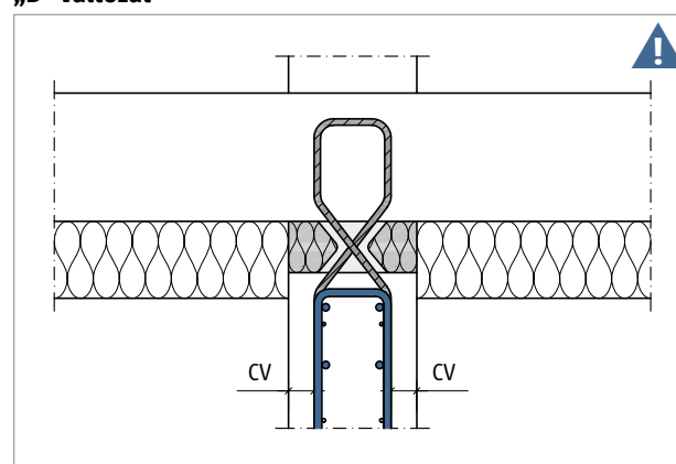
Ábra 120: Schöck Sconnex® W-N-VH típus: „B” változat (kis falvastagság esetén) – helyszíni vasalás; a fal hosszvasalása a Schöck Sconnex® nyíróvasain belül halad (nem támasztja meg kívülről)
