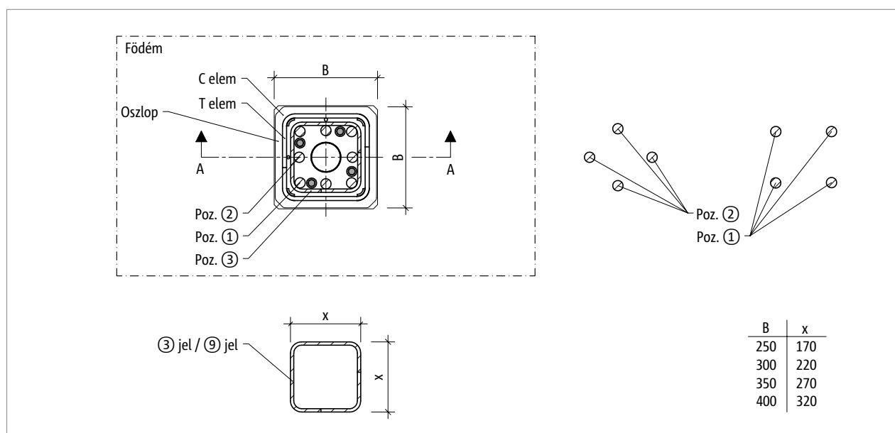
Ábra 82: Schöck Sconnex® P típus: helyszíni vasalás az oszlop keresztmetszetében
