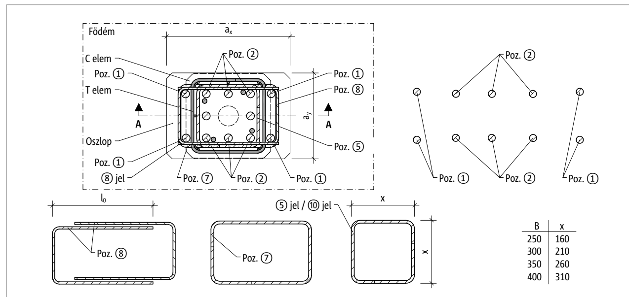
Ábra 88: Schöck Sconnex® P típus: helyszíni vasalás az oszlop keresztmetszetében
