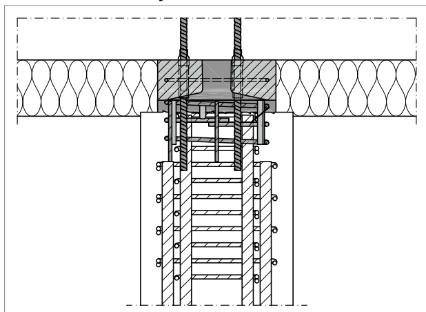
Ábra 77: Schöck Sconnex® P típus: vasalás a 2. tartományban – oszlop hosszanti metszet
