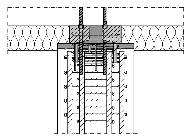
Ábra 79: Schöck Sconnex® P típus: vasalás a 3. tartományban – oszlop hosszanti metszet
