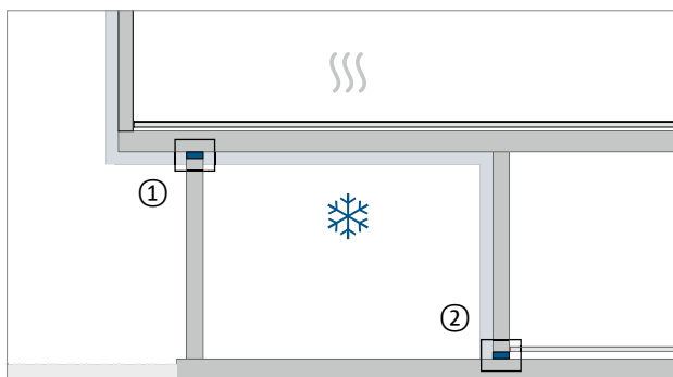
Ábra 3: Külső oszlop és mélygarázsfallal Schöck Sconnex® elemmel
