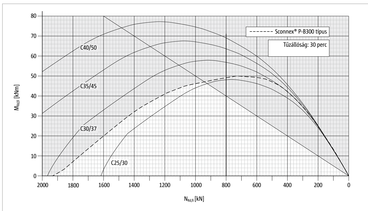
Ábra 44: Schöck Sconnex® P-B300 típus: interakciós ábra tűzesetre történő méretezéshez; R 30-as tűzállósági osztály
