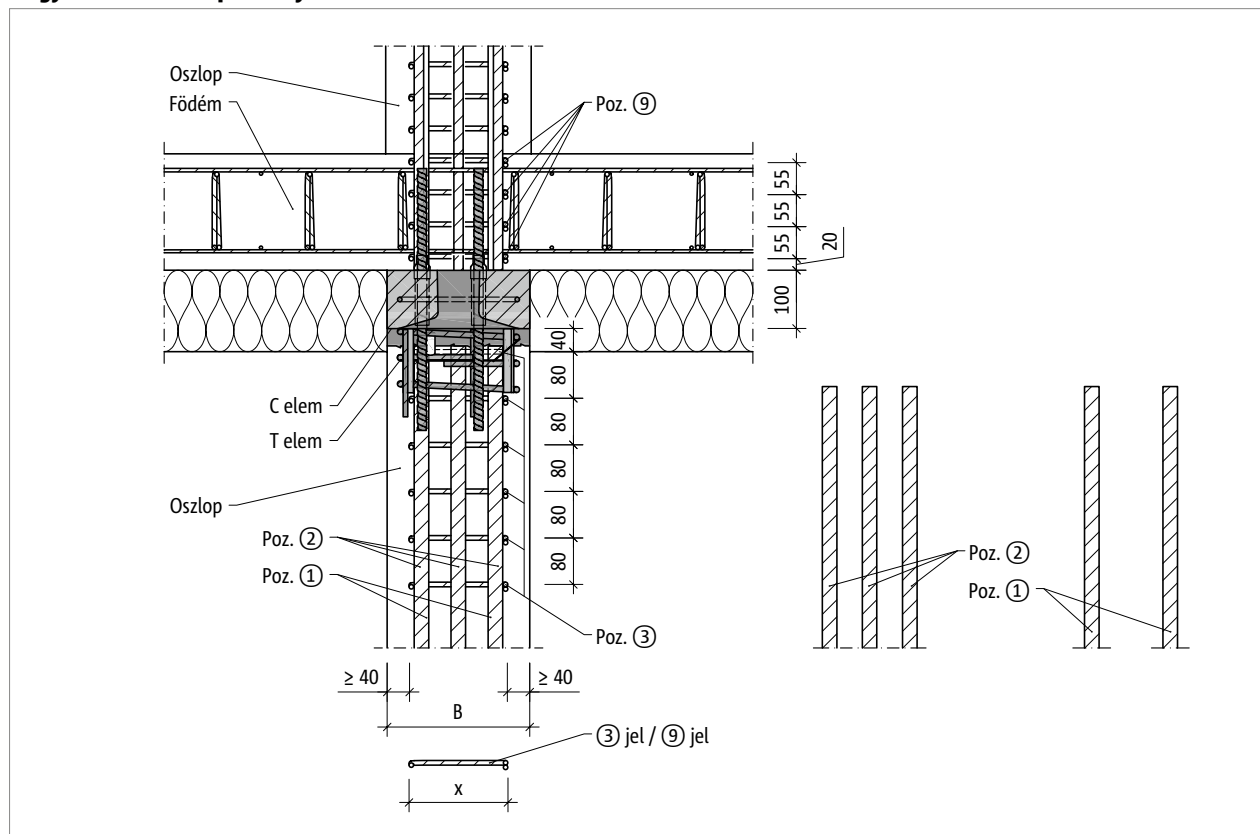
Ábra 81: Schöck Sconnex® P típus: helyszíni vasalás az oszlop A-A hosszmeteszetében
