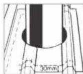
3. Rajzolja fel a Dektite vízzáró gumiharang kontúrját a tetőn. Távoltítsa el a gumiharangot és jelöljön fel 30 mm-es ráartást.
