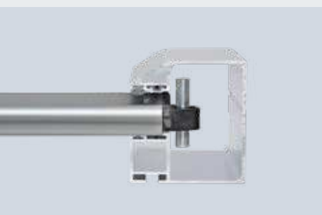
DD redőnykapu Decotherm S profil acél viharkapoccsal (7500 mm-es kapuszélességtől ill. -magasságtól vagy opcionálisan nagyobb szélterhelési követelményhez)
