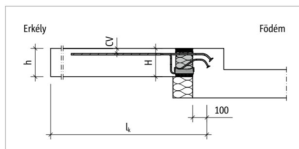
Ábra 84: Schöck Isokorb® XT KL-O típus: Statikai rendszer
