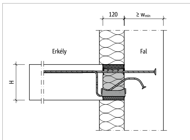
Ábra 76: Schöck Isokorb® XT KL-U típus: Felső fal csatlakozás külső szigetelésnél
