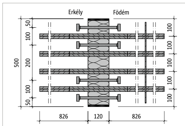
Ábra 163: Schöck Isokorb® XT QP-VV9 típus: termék alaprajz
