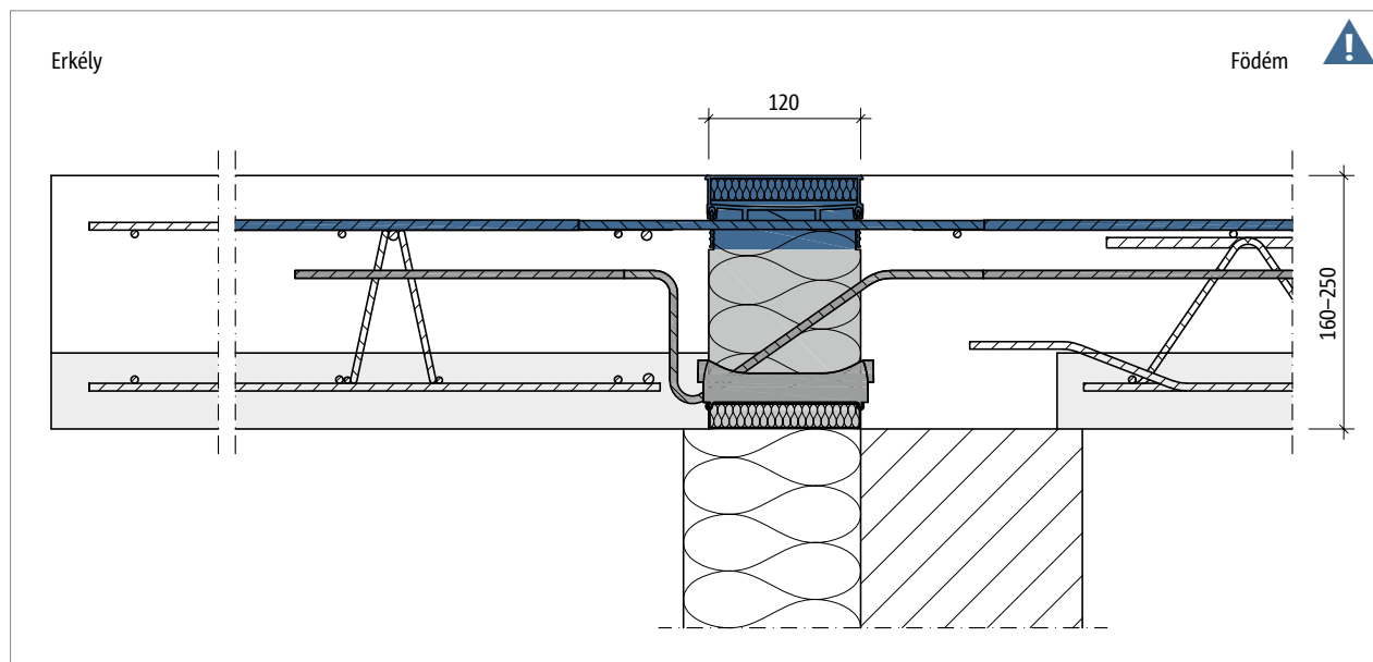
Ábra 68: Schöck Isokorb® XT KL-F típus: A felső rész a húzóerő átadásához szükséges
