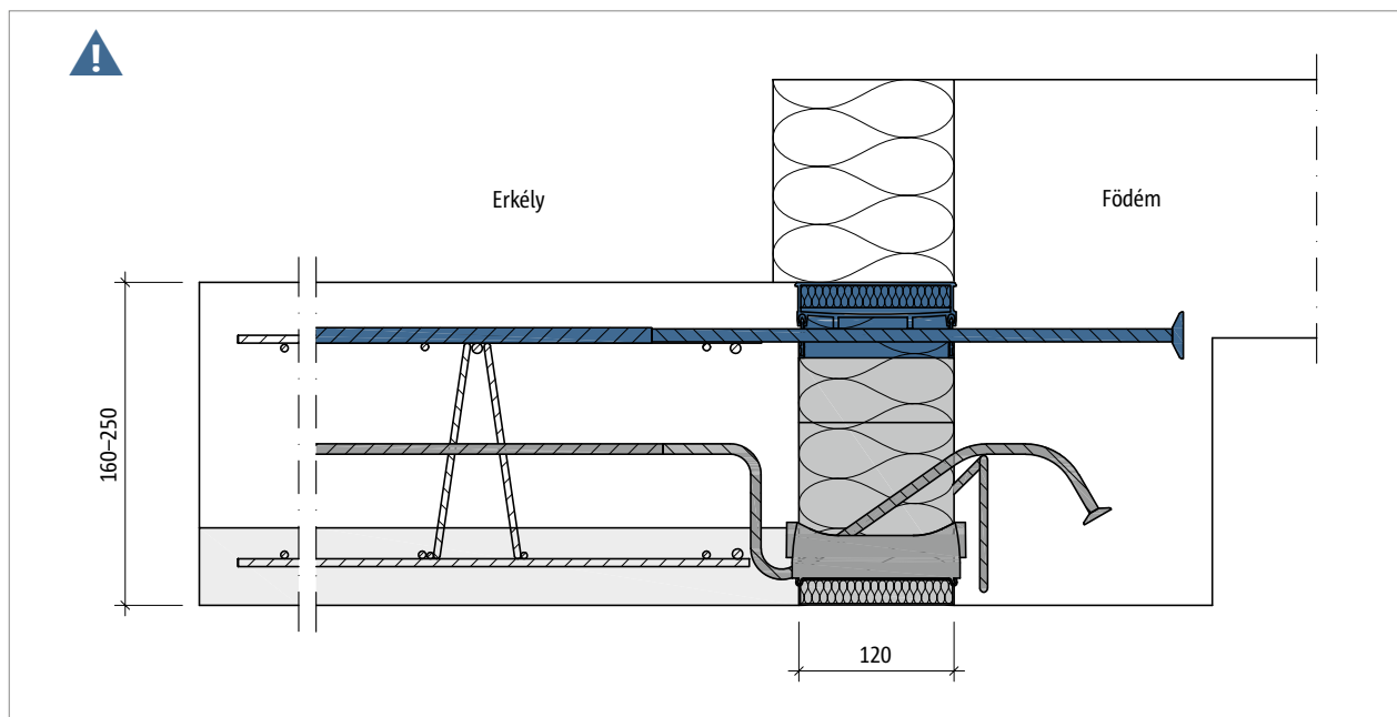
Ábra 116: Schöck Isokorb® XT KL-U-F típus: felső részből, (opcionális) közdarabból és alsó részből álló többrészes felépítés. Itt: a felső rész színnel jelölt.
