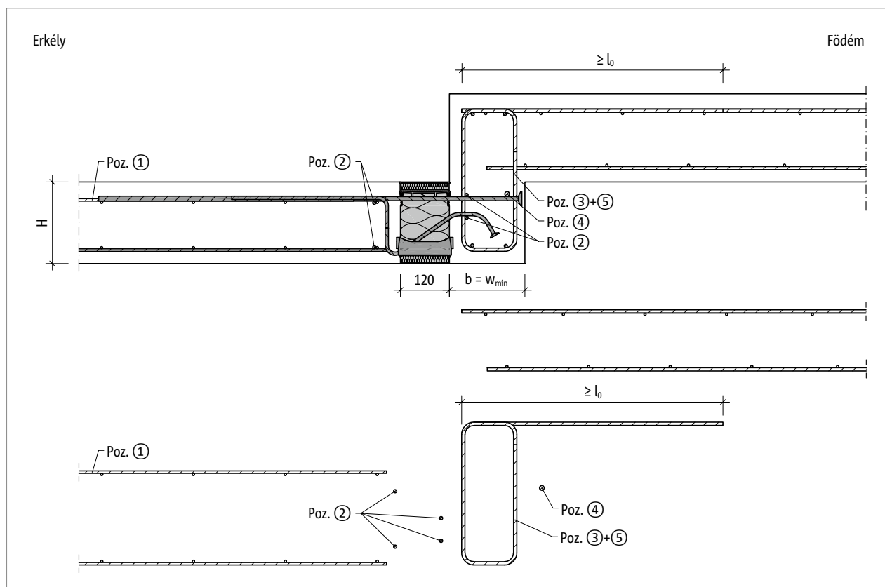
Ábra 94: Schöck Isokorb® XT KL-U típus: Helyszíni vasalás - erkély lefelé födémugrással, minimális szerkezeti elemmérettel ( w_{tényl} = w_{min} )
