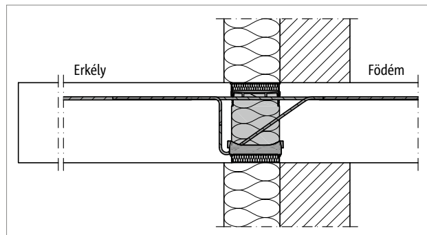
Ábra 23: Schöck Isokorb® XT KL típus: Csatlakozás hőszigetelő rendszernél
