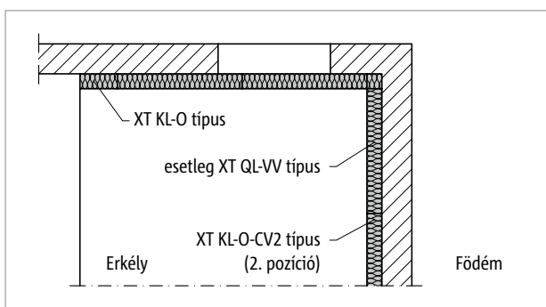
Ábra 73: Schöck Isokorb® XT KL-O, XT QL-VV típusok: Két oldalon felfekvő erkély belső sarokban
