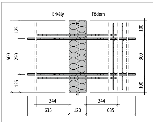
Ábra 229: Schöck Isokorb® XT DP-MM1-VV1 típus: alaprajz
