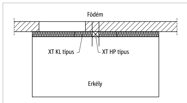
Ábra 19: Schöck Isokorb® XT KL típus: Konzolosan kinyúló erkély; opcionálisan XT HP típussal terv szerinti vízszintesen ható erők esetén (pl. zárt mellvédek)
