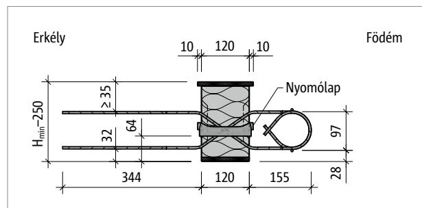
Ábra 132: Schöck Isokorb® XT QL-VV1 – QL-VV4 típus: termékmetszet
