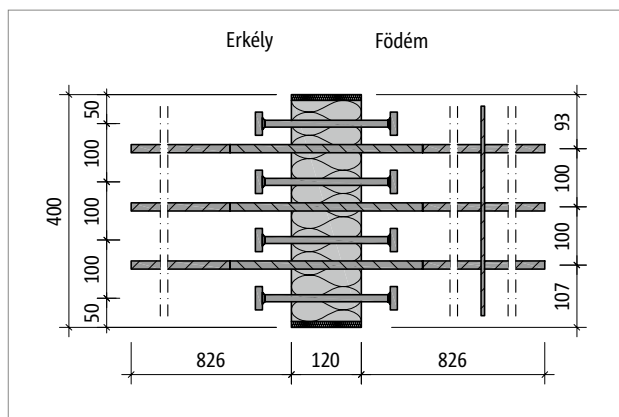
Ábra 162: Schöck Isokorb® XT QP-V8 típus: termék alaprajz
