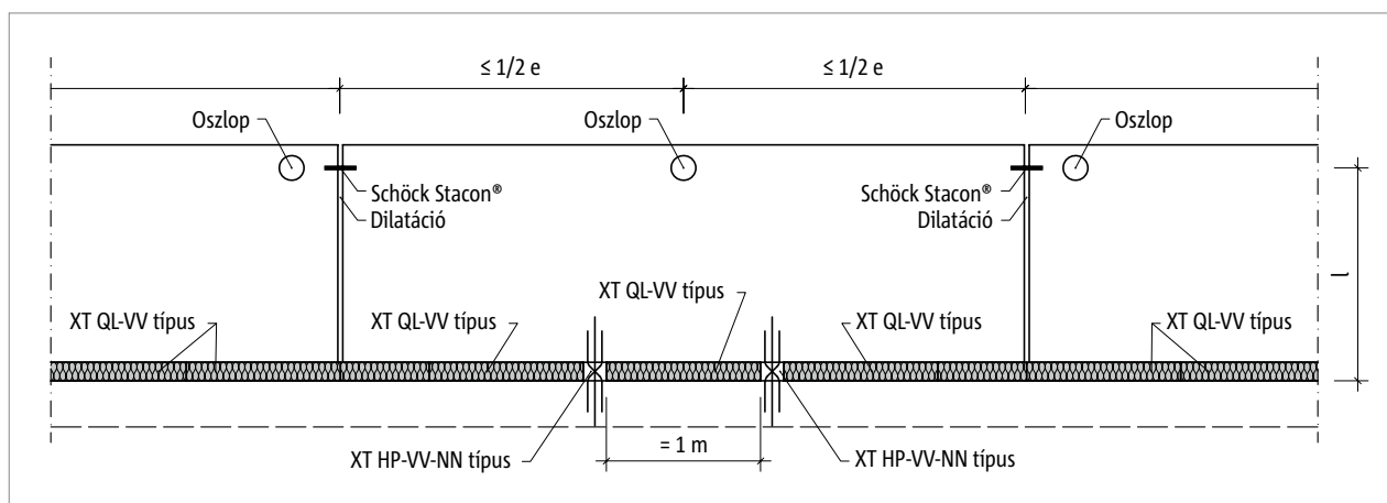
Ábra 17: Schöck Isokorb® XT HP típus: Dilatációs hézagok elrendezése
