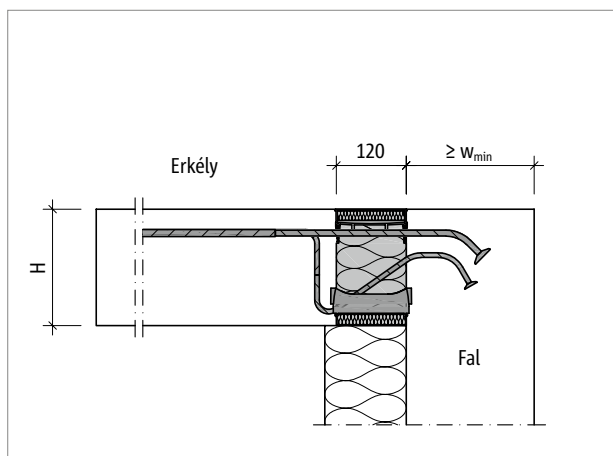
Ábra 79: Schöck Isokorb® XT KL-O típus: Alsó fal csatlakozás külső szigetelésnél
