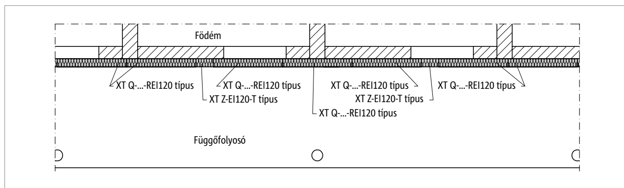
Ábra 1: Schöck Isokorb® XT QL-...-REI120 típus, XT ZL-EI120 típus : Tűzhatároló függőfolyosó
