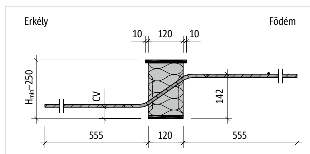
Ábra 159: Schöck Isokorb® XT QP-Z-V1 – QP-Z-V3 típus: termékmetset
