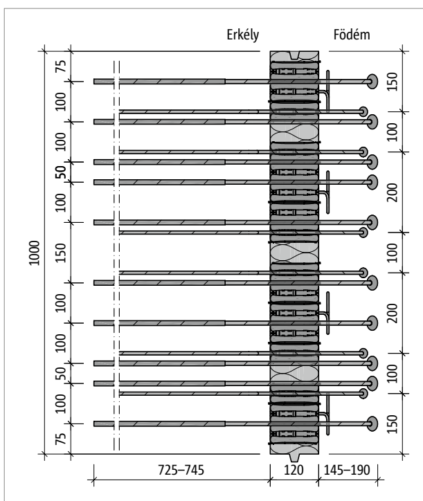
Ábra 92: Schöck Isokorb® XT KL-O-M4 típus: termékcalaprajz
