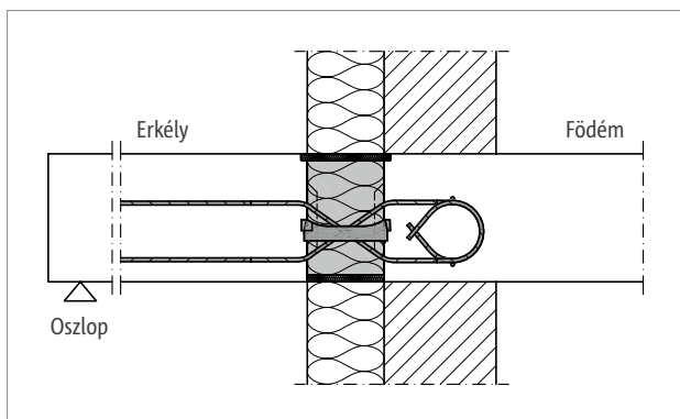
Ábra 121: Schöck Isokorb® XT QL-VV típus: Csatlakozás hőszigetelő rendszer-nél
