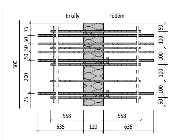
Ábra 193: Schöck Isokorb® XT CL-L-M1-V1 típus: termékábráj
