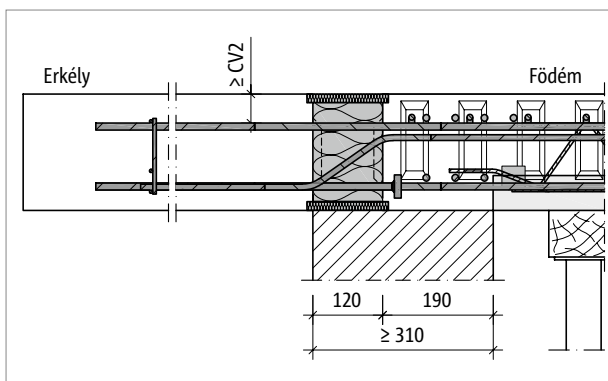
Ábra 202: Schöck Isokorb® XT CL típus: kéregpaneles erkély peremalátámasztással, hőszigetelő falazattal (XT CL-R-CV2 típus metszete, CL-L-CV1 típus nézete)
