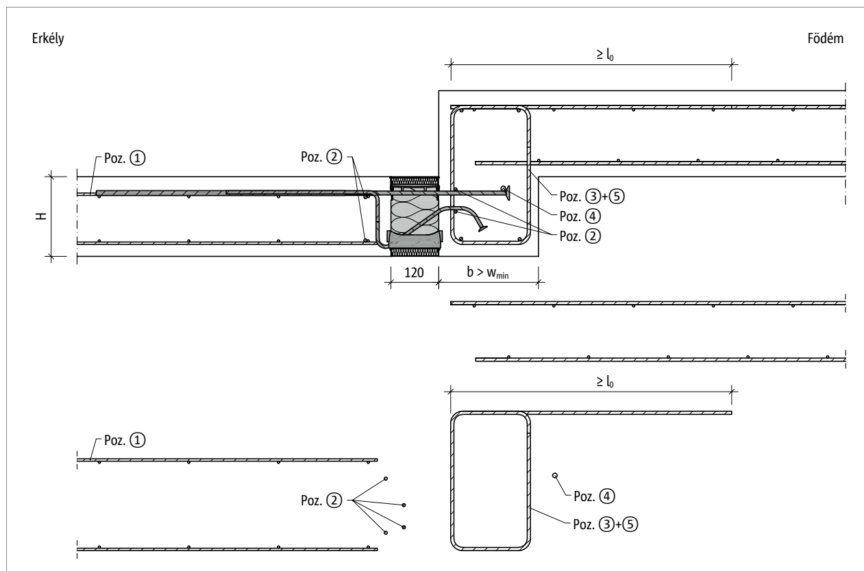
Ábra 95: Schöck Isokorb® XT KL-U típus: Helyszíni vasalás - erkély lefelé födémugrással, nagyobb építőelem mérettel ( w_{tényl} > w_{min} )
