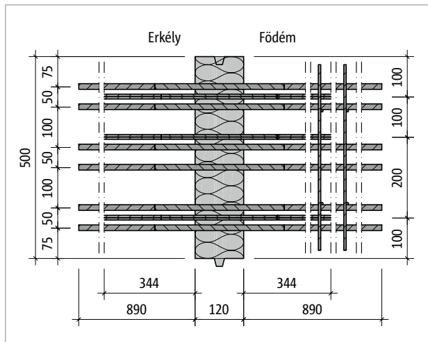
Ábra 232: Schöck Isokorb® XT DP-MM6-VV1 típus: alaprajz
