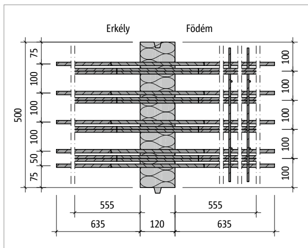
Ábra 230: Schöck Isokorb® XT DP-MM4-VV4 típus: alaprajz
