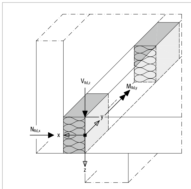
Ábra 242: Előjel szabály Schöck Isokorb® XT AP típus számításához, földem-perem elé helyezett mellvéd esetén
