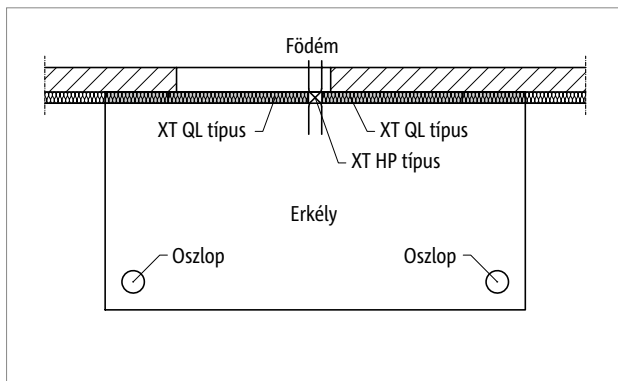
Ábra 117: Schöck Isokorb® XT QL típus: Oszloppal alátámasztott erkély
