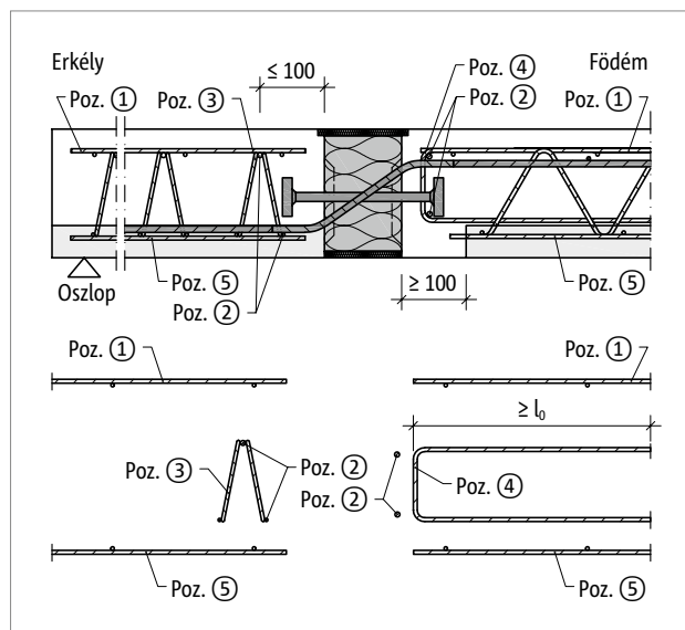
Ábra 166: Schöck Isokorb® XT QP típus: Helyszíni vasalás rácsos borda esetén
