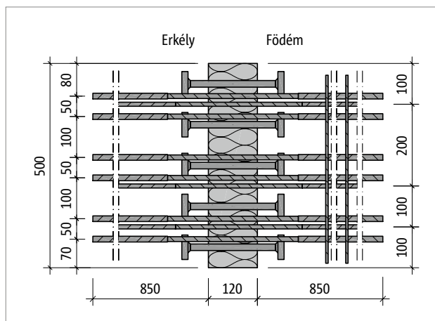
Ábra 44: Schöck Isokorb® XT KP-M11 típus: termékalaprajz
