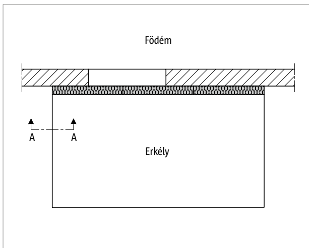
Ábra 49: Schöck Isokorb® XT KL, KP típus: Konzolos erkély
