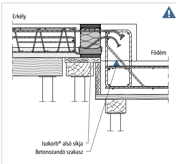
Ábra 115: Schöck Isokorb® XT KL-O-F típus: erkély kéregpanellel felső magasságtolással
