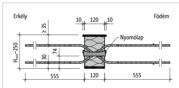
Ábra 133: Schöck Isokorb® XT QL-VV6 – QL-VV8 típus: termékmetszet
