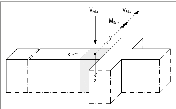
Ábra 262: Schöck Isokorb® XT WL típus: Előjel szabály a méretezéshez
