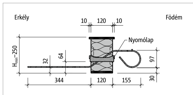
Ábra 127: Schöck Isokorb® XT QL-V1 – QL-V4 típus: termékmetszet
