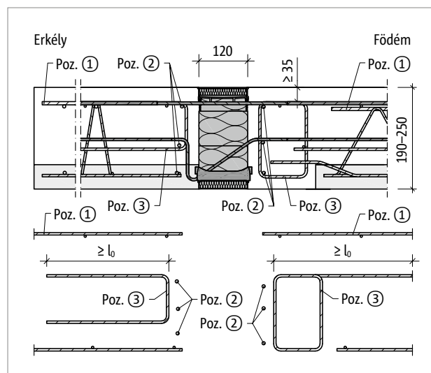
Ábra 64: Schöck Isokorb® XT KL-F típus: Helyszíni vasalás h = 190-250 mm erkélylemez vastagságánál
