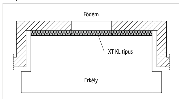
Ábra 21: Schöck Isokorb® XT KL típus: Erkély beugró homlokzaton
