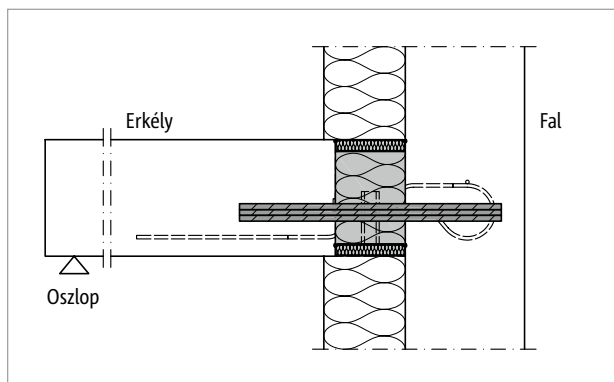
Ábra 208: Schöck Isokorb® XT QL HP-VV-NN típus: Csatlakozás külső hőszigetelésű vasbeton falhoz
