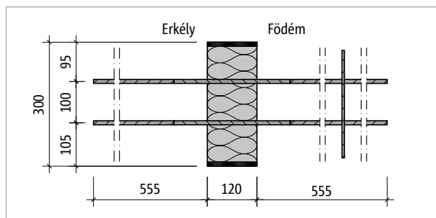
Ábra 161: Schöck Isokorb® XT QP-Z-V1 típus: termék alaprajz
