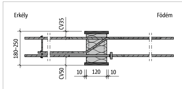
Ábra 191: Schöck Isokorb® XT CL-L-CV1 típus: termékmetszet
