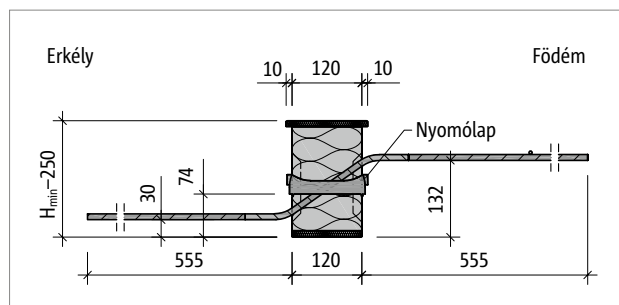
Ábra 129: Schöck Isokorb® XT QL-V6 – QL-V8 típus: termékmetszet
