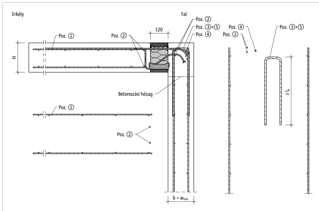
Ábra 100: Schöck Isokorb® XT KL-O: helyszíni vasalás minimális falvastagság és alsó falcsatlakozás esetén ( w_{\text{megl}} = w_{\text{min}} )
