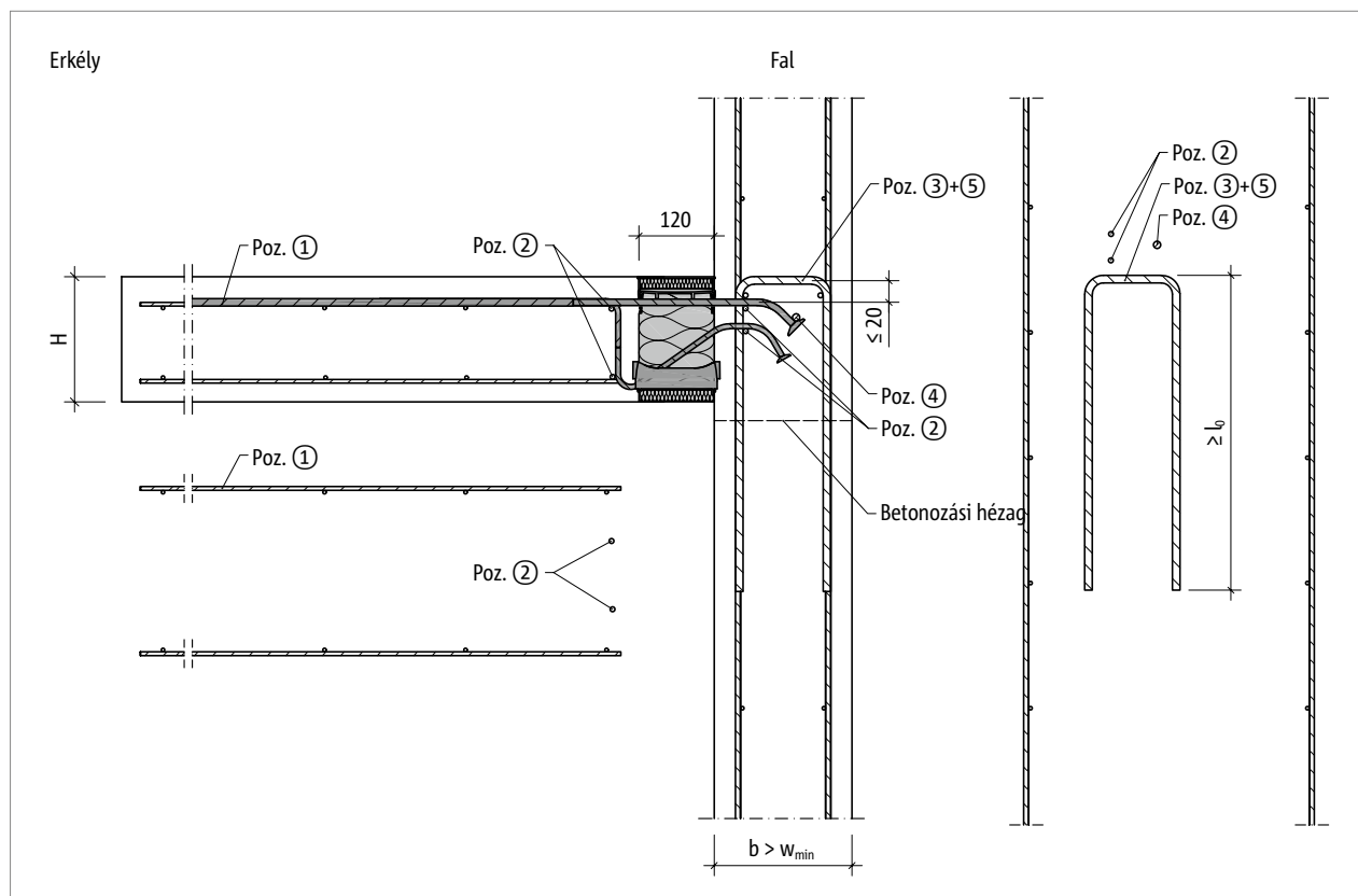
Ábra 101: Schöck Isokorb® XT KL-O típus: Helyszíni vasalás - falcsatlakozás nagyobb szerkezeti elemmérettel ( w_{\text{tényl}} > w_{\text{min}} )
