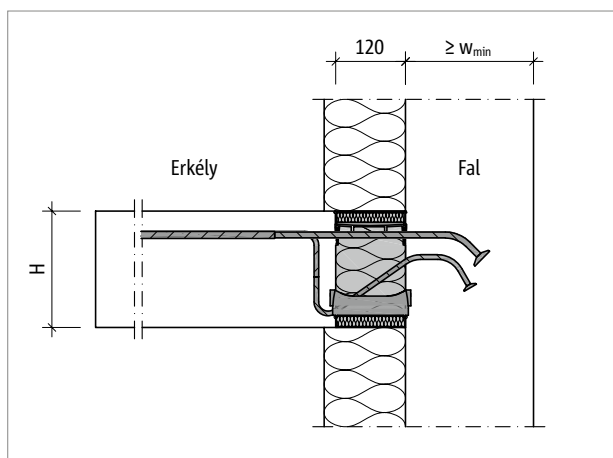
Ábra 77: Schöck Isokorb® XT KL-O típus: Alsó fal csatlakozás külső szigetelésnél
