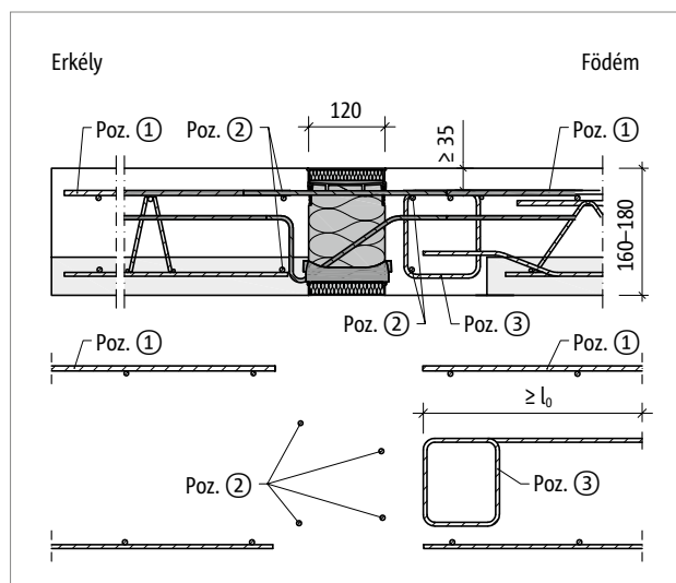
Ábra 63: Schöck Isokorb® XT KL-F típus: Helyszíni vasalás h = 160-180 mm erkélylemez vastagságánál
