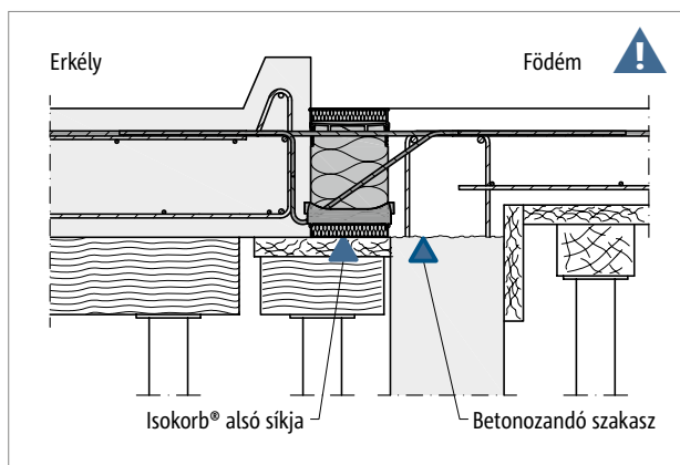
Ábra 54: Schöck Isokorb® XT KL típus: Teljes keresztmetszetben előregyártott erkély magasságeltolós födémmel előregyártott vasbeton falon
