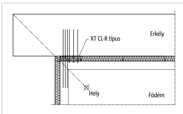
Ábra 184: Schöck Isokorb® XT CL típus: épületsarkon túlnyúló erkély (XT CL-R típus felhasználásával)
