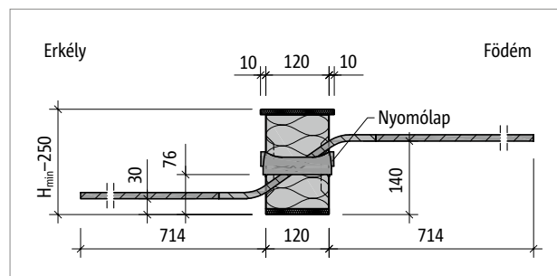
Ábra 130: Schöck Isokorb® XT QL-V10 típus: termékmetszet
