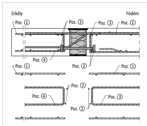
Ábra 50: Schöck Isokorb® XT KP-M11 típus: Helyszíni vasalás közzetett alátámasztás esetén
