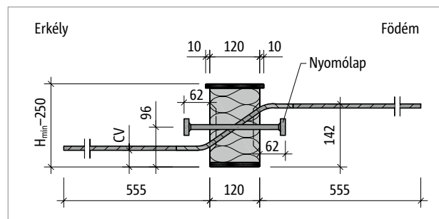
Ábra 153: Schöck Isokorb® XT QP-V2 típus: termékmetset
