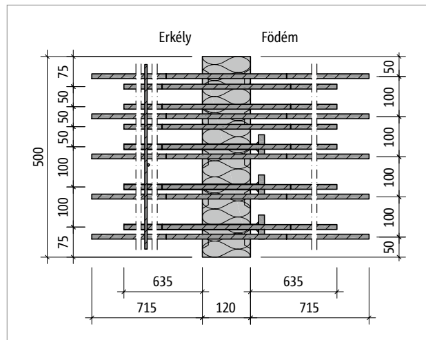
Ábra 195: Schöck Isokorb® XT CL-L-M2-V2 típus: termékábráj
