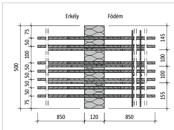
Ábra 45: Schöck Isokorb® XT KP-M12 típus: termékalaprajz
