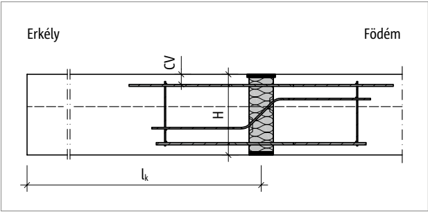
Ábra 255: Schöck Isokorb® XT BP típus: Statikai rendszer
