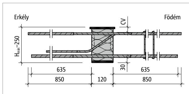
Ábra 43: Schöck Isokorb® XT KP-M12 – KL-M13 típus: termékmetset
