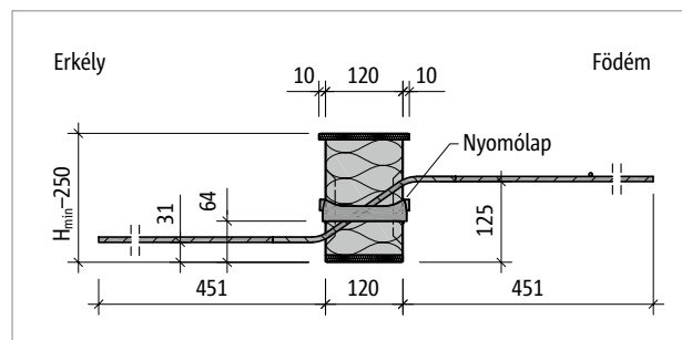
Ábra 128: Schöck Isokorb® XT QL-V5 típus: termékmetszet
