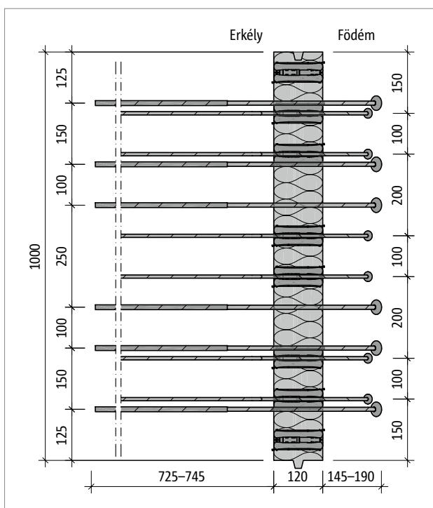
Ábra 91: Schöck Isokorb® XT KL-O-M2 típus: termékcalaprajz
