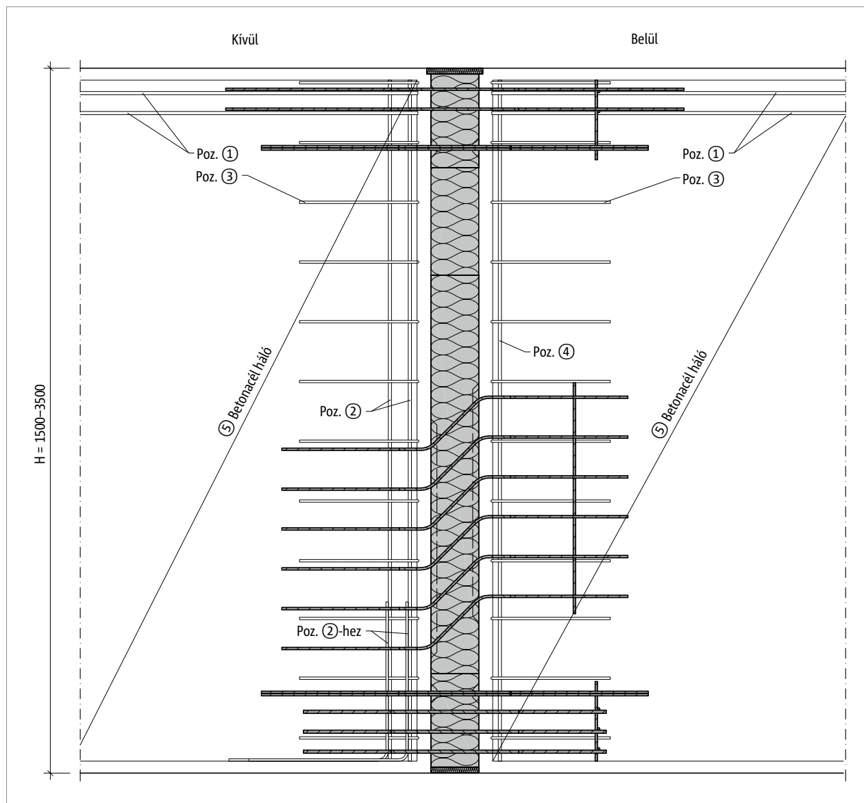
Ábra 269: Schöck Isokorb® XT WL típus: Helyszíni vasalás; metszet
