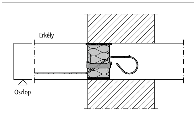
Ábra 119: Schöck Isokorb® XT QL típus: Csatlakozás egyhéjú, homogén hőszigetelt falazat esetén (XT QL-V1 típustól XT QL-V4 típusig)
