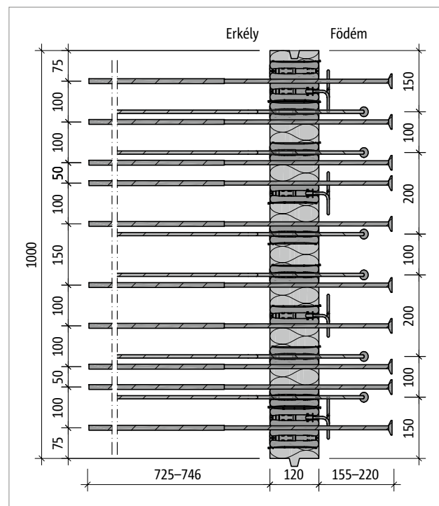
Ábra 88: Schöck Isokorb® XT KL-U-M4 típus: termék alaprajz
