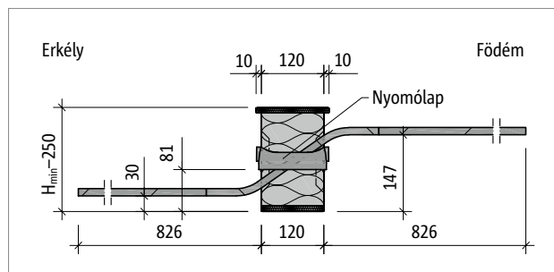
Ábra 131: Schöck Isokorb® XT QL-V11 típus: termékmetszet
