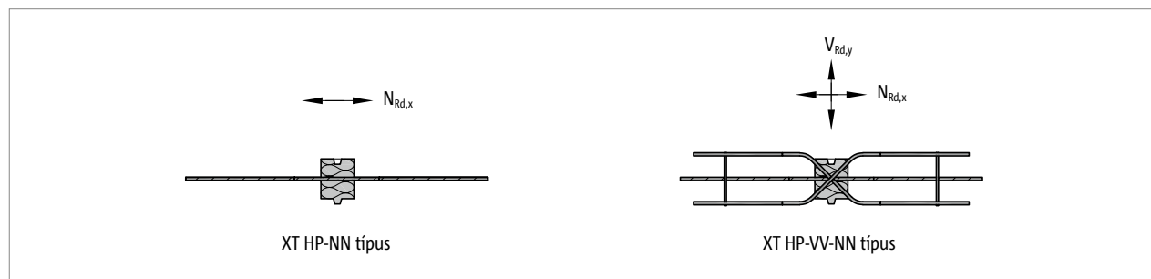
Ábra 209: Schöck Isokorb® XT HP típus: Típus kiválasztása
