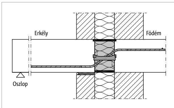
Ábra 120: Schöck Isokorb® XT QL típus: Csatlakozás magszigetelt kéthéjú falazatnál (XT QL-V5 típustól XT QL-V8 típusig)
