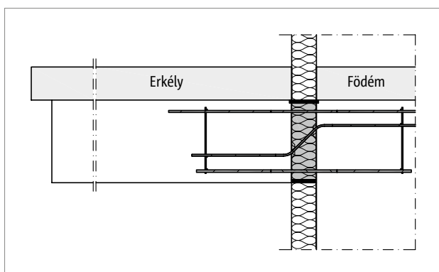
Ábra 253: Schöck Isokorb® XT BP típus: Erkélyszerkezet konzolosan túlnyúló gerendákkal (előregyártott erkély)
