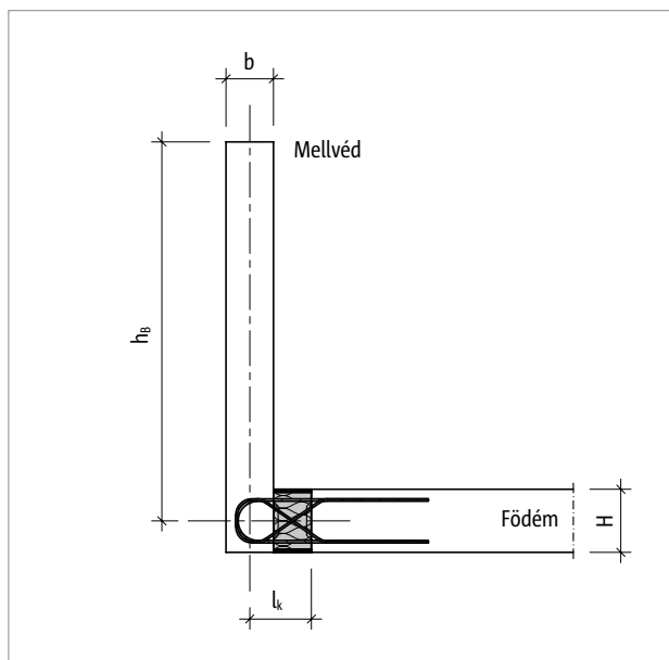
Ábra 244: Schöck Isokorb® XT AP típus: Statikai modell, mellvédmagasság: h_B
