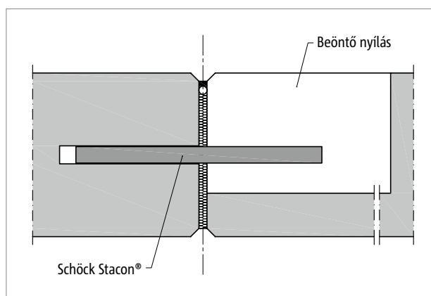
Ábra 15: Schöck Stacon®: Dilatációs hézag kialakítása, előregyártott erkély elemek esetén
