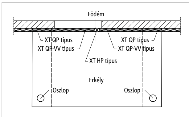
Ábra 118: Schöck Isokorb® XT QP, QL-VV típus: Oszloppal alátámasztott erkély, csatlakozás különböző alátámasztási merevséggel; opcionálisan XT HP típus a terv szerinti vízszintes erő továbbítására
