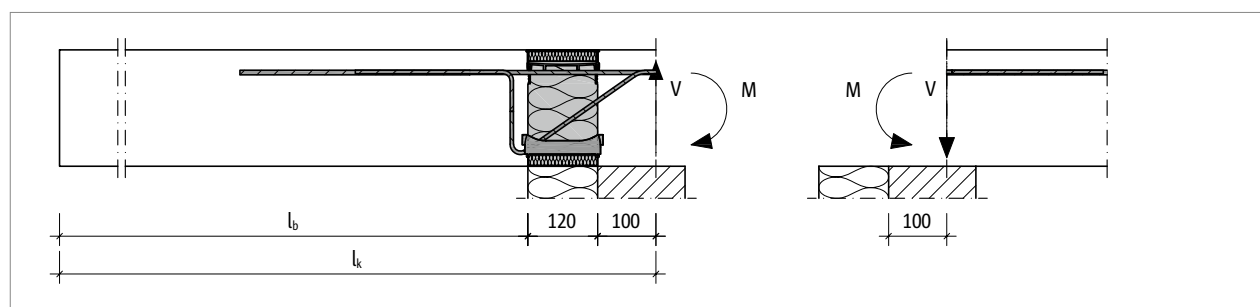
Ábra 9: Schöck Isokorb® XT KL típus: A födémlemezzen feltételezett, számított méretezési keresztmetszeti igénybevétel
