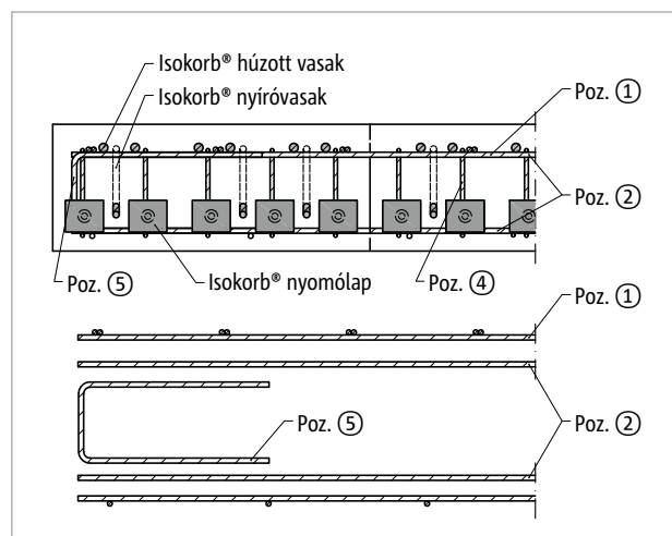
Ábra 51: Schöck Isokorb® XT KP-M11 típus: erkélyoldali helyszíni vasalás A-A metszete; Poz. 5 = konstruktív peremvasalás a szabad perem mentén
