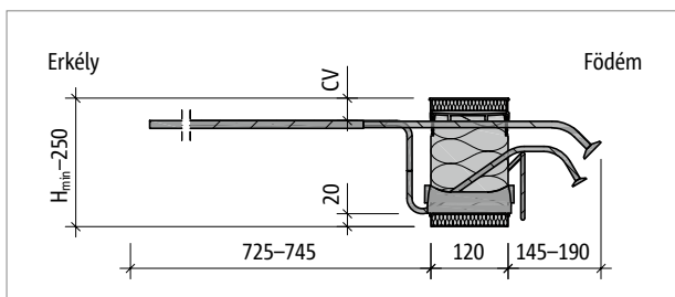
Ábra 90: Schöck Isokorb® XT K-O-M4 típus: Metszet
