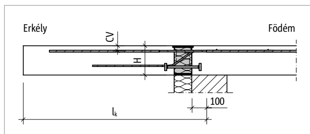
Ábra 28: Schöck Isokorb® XT KP-M11 típus: Statikai váz
