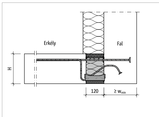
Ábra 78: Schöck Isokorb® XT KL-U típus: Felső fal csatlakozás külső szigetelésnél
