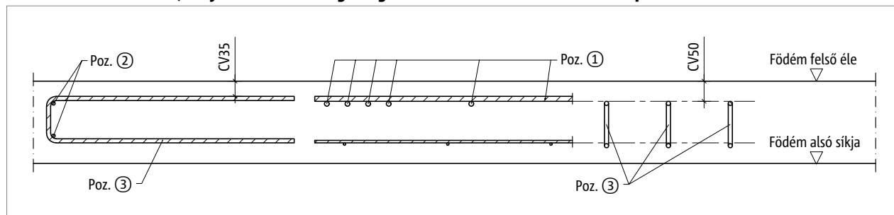
Ábra 197: Schöck Isokorb® XT CL típus: Külső sarok helyszíni vasalása (XT CL-L-CV1 metszeti rajz, XT CL-R-CV2 nézeti rajz)
