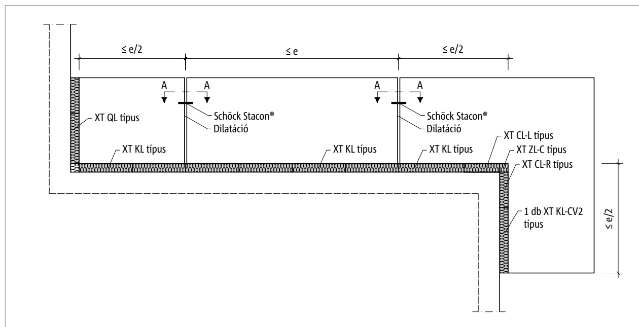
Ábra 13: Schöck Isokorb® XT KL típus: Dilatációs hézag kialakítása tengely irányú dilatációra képes nyíróerőtűskével pl. Schöck Stacon®
