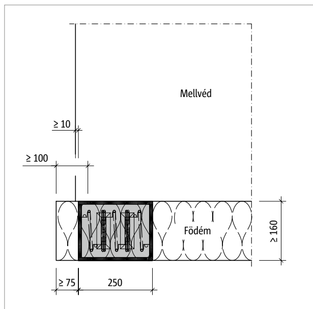
Ábra 246: Schöck Isokorb® XT AP típus, vízszintes elhelyezés: Peremtávolságok, nézet
