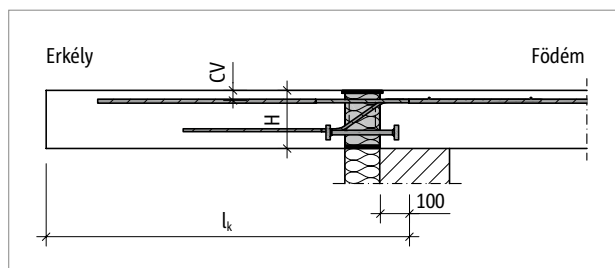
Ábra 31: Schöck Isokorb® XT KP-M11 típus: Statikai váz
