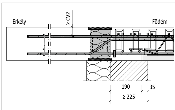
Ábra 200: Schöck Isokorb® XT CL típus: kéregpaneles erkély peremalátámasztás nélkül, homlokzati hőszigetelő rendszerrel (XT CL-R-CV2 típus metszete, CL-L-CV1 típus nézete)
