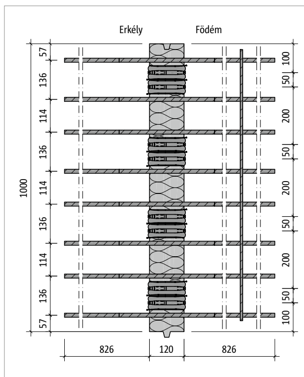
Ábra 135: Schöck Isokorb® XT QL-V11 típus: termék alaprajz
