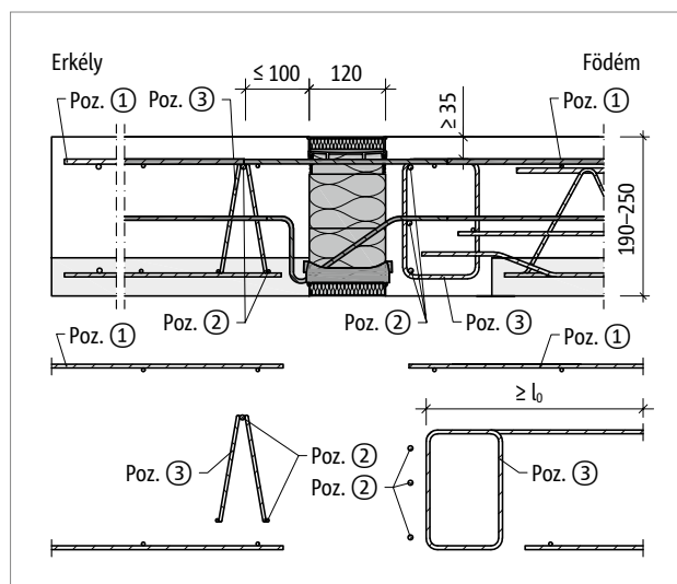
Ábra 65: Schöck Isokorb® XT KL-F típus: Helyszíni vasalás h = 190-250 mm erkélylemez vastagságánál, rácstartóval
