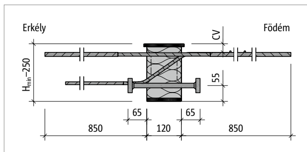
Ábra 42: Schöck Isokorb® XT KP-M11 típus: termékmetset
