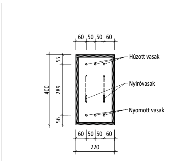
Ábra 257: Schöck Isokorb® XT BP típus: terméknézet
