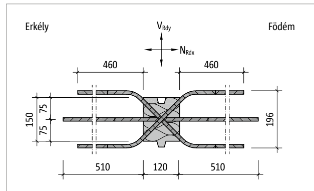
Ábra 218: Schöck Isokorb® XT HP-VV2-NN1 típus: Felső metszete
