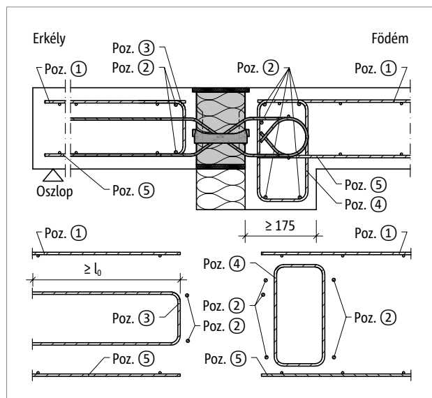
Ábra 138: Schöck Isokorb® XT QL-VV1 – VV4: helyszíni vasalás alulborda esetén
