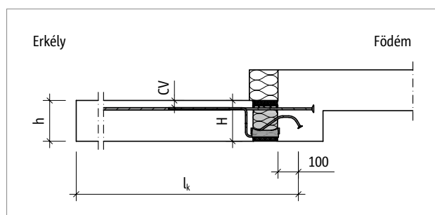
Ábra 83: Schöck Isokorb® XT KL-U típus: Statikai rendszer
