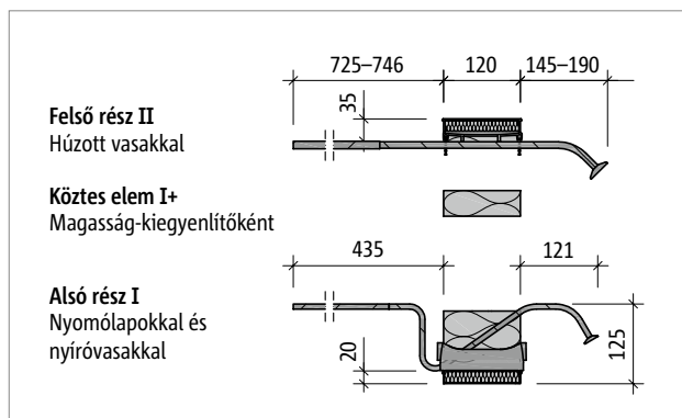
Ábra 106: Schöck Isokorb® XT KL-O-F-M1-V1-CV1 típustól KL-O-F-M3-V1-CV1 típusig
