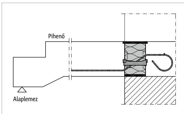
Ábra 122: Schöck Isokorb® XT Typ QL típus: Lépcsőpihenő csatlakozása egyhéjú, homogén hőszigetelő falazat esetén (XT QL-V1 típustól XT QL-V4 típusig)
