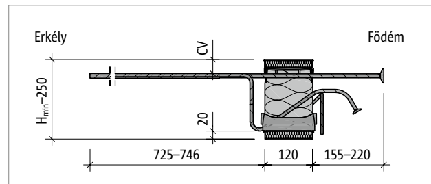
Ábra 86: Schöck Isokorb® XT K-U-M4 típus: Metszet
