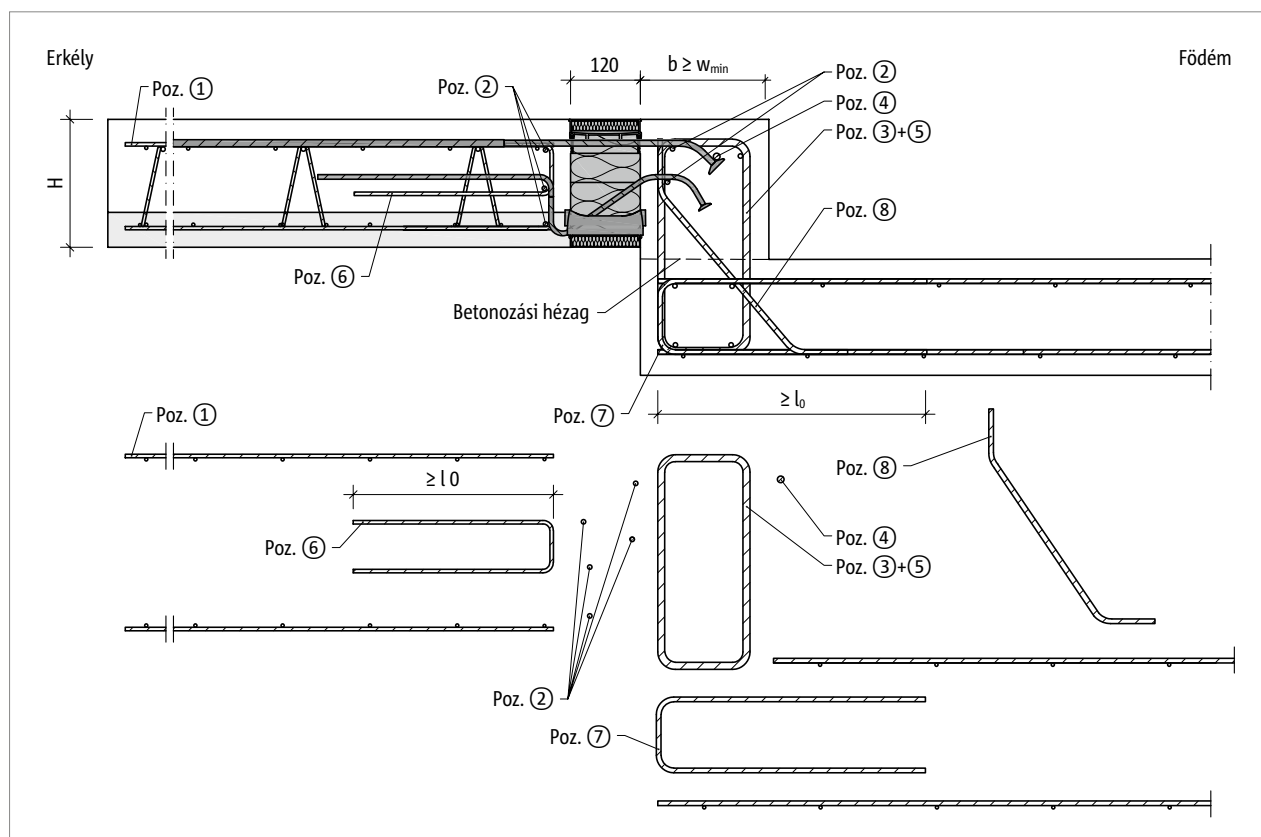
Ábra 110: Schöck Isokorb® XT KL-O-F típus: Helyszíni vasalás, felfelé földmugrásos erkély
