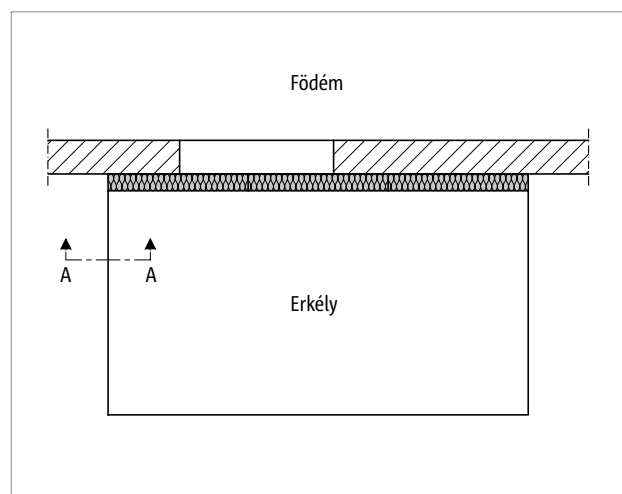
Ábra 52: Schöck Isokorb® XT KL, KP típus: Konzolos erkély
