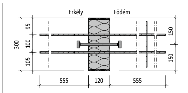
Ábra 160: Schöck Isokorb® XT QP-V1 típus: termék alaprajz
