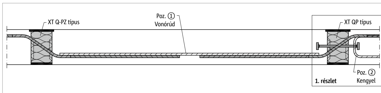
Ábra 170: Schöck Isokorb® XT QP-Z, QP típus: A-A metszet; vasalás csatlakozása – húzott borda
