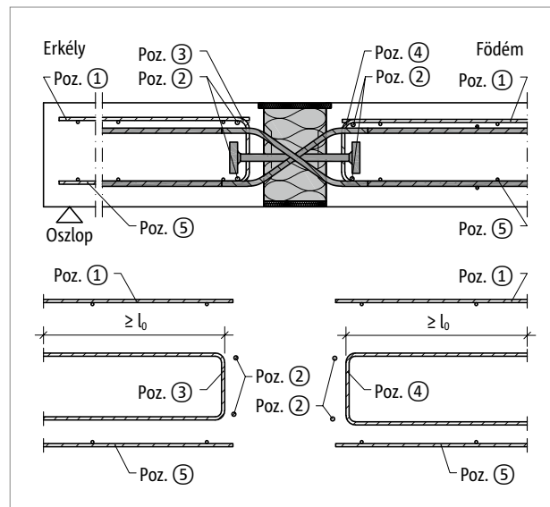
Ábra 165: Schöck Isokorb® XT QP-VV típus: helyszíni vasalás
