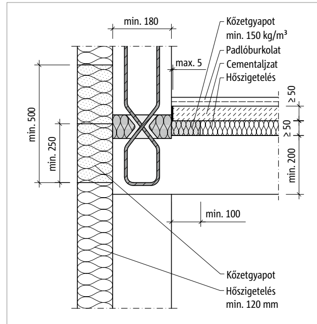
Ábra 136: Schöck Sconnex® W típus: gyúlékony (külső) homlokzati hőszigetelő rendszer esetén, kőzetgyapot tűzvédelmi sávval és szegélyszárral a lépéshang szigetelés síkjában
