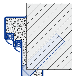
Saroktok (duplafalcos tok) Szerelőfüles rögzítés
