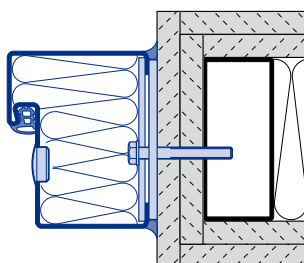
Blokktok 95 / 75 mm Csavaros szerelés
