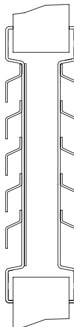
Szellőzőrács
