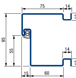
Blokktok 95 / 75 mm, egyedi, árnyékhoronnyal
