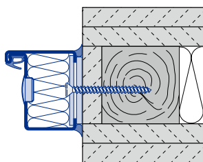
Blokktok 62 / 55 mm Csavaros szerelés
