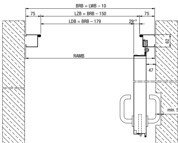
Blokkok, 62 / 75 (STU)
