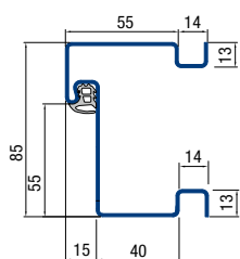
Blokktok 85 / 55 mm egyedi, árnyékhoronnyal
