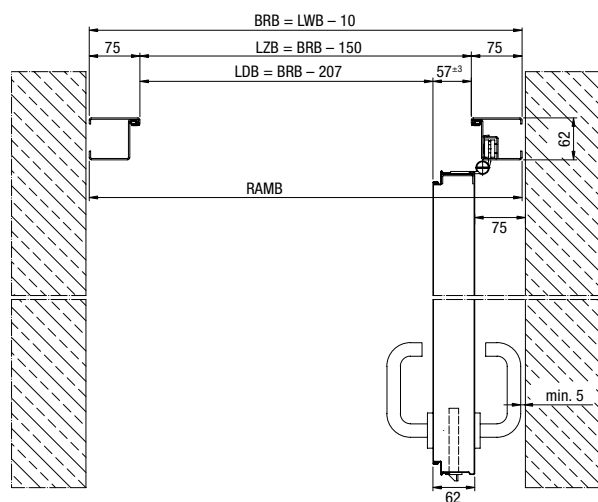
Blokktok, 62 / 75 (STS)
