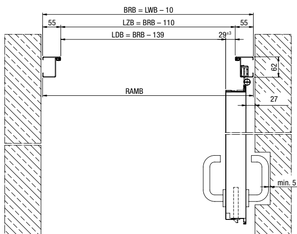
Blokkok, 62 / 55 (STU)
