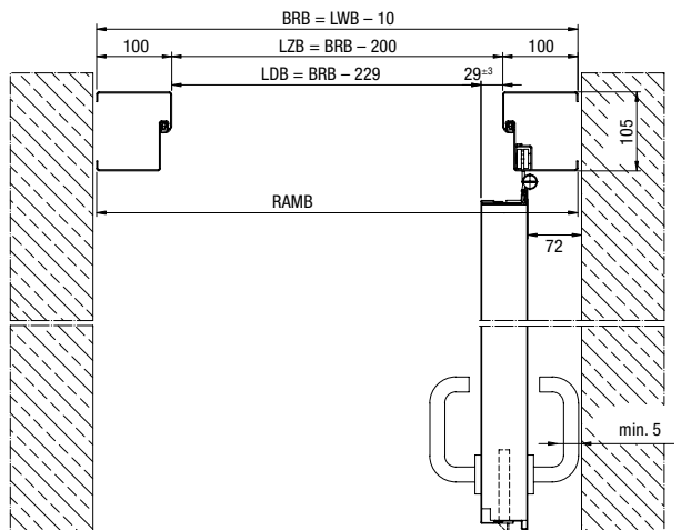
Blokkok, 105 / 100 (STU)
