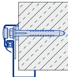
Saroktok 20, egyedi Tiplis rögzítés (Standard)
