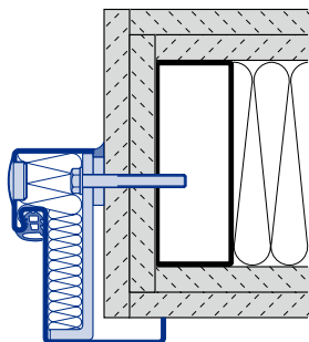
Saroktok 40 (standard) Csavaros szerelés
