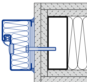
Blokktok 95 / 55 mm Csavaros szerelés
