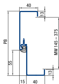
Befoglalótok 40, 2-részes
