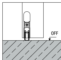
Hidraulikusan süllyeszthető padlótömítés
