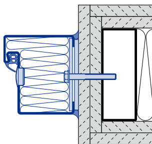
Blokktok 85 / 75 mm (standard) Csavaros szerelés
