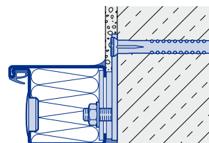
Blokkok 62 / 75 mm Tiplis rögzítés (téglafal) fallal egy síkot alkotó szerelés, 95-ös horgonylemez, elvakolva Pántoldal
