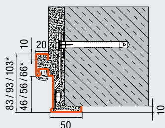
Saroktok, tiplis rögzítéssel a falkávéban (tégla fal / betonfal)
