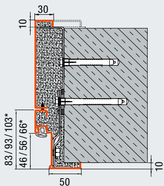
Sarok- és kiegészítőtok, rejtett tiplis rögzítéssel és hegesztett szerelésű kiegészítőtokokkal (Nem vakolt tégla fal / betonfal)
