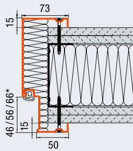
Befoglalók, csavaros szereléssel (szerelt fal)
