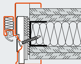
Átlós rögzítés Vario B53 kiegészítőtokkal, 2-héjű befoglalótokként (F90 A szerelt fal)
