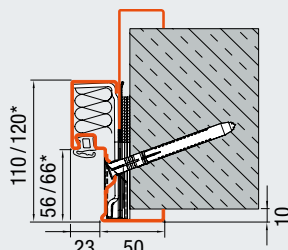
VarioFix Fire (tégla fal / betonfal)
