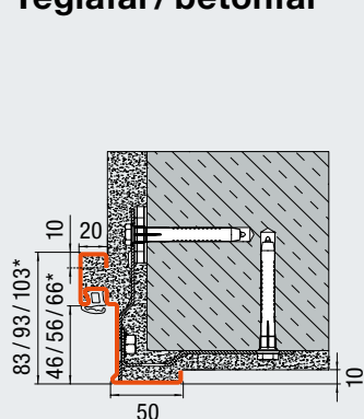
Saroktok, tiplis rögzítéssel (tégla fal / betonfal)
