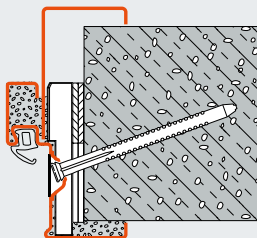
Átlós rögzítés Vario B53 kiegészítőtokkal, 2-héjű befoglalótokként (gázbeton fal)
