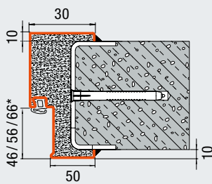
Befoglalók, hegesztett szereléssel (gázbeton fal)
