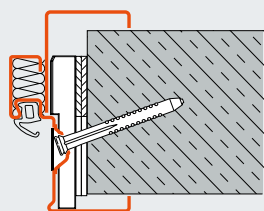
Átlós rögzítés Vario B53 kiegészítőtokkal, 2-héjű befoglalótokként (Nem vakolt téglafal / betonfal)
