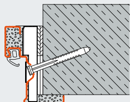
Átlós rögzítés (Nem vakolt téglafal / betonfal)
