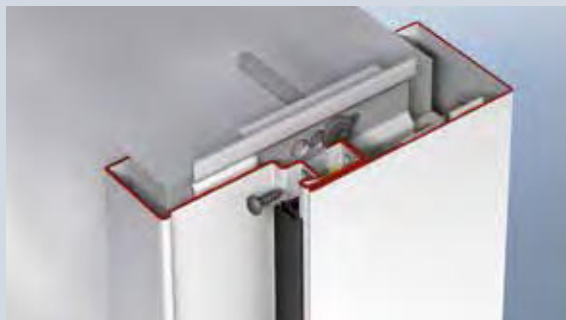
Csavarozza a 2. ellentokprofilát a tömítési hornyon keresztül az 1. tokprofilhoz, majd takarja el azt az ajtó tömítéssel
