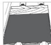
4. A 30 mm-es vonalon belül vágja ki a tetőt. Sorjázza le az éles széleket. A tetőkivágás stabilitásához, ahol szükséges, szereljük fel a kíváltó gerendákat.
