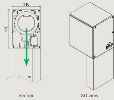
Fixscreen® 100 Slim - IM 7A - Head box
