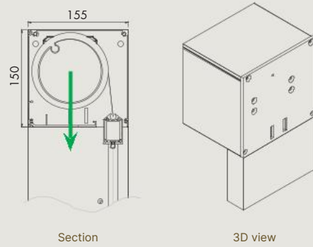
Fixscreen® 150 - IM 7A - Head box
