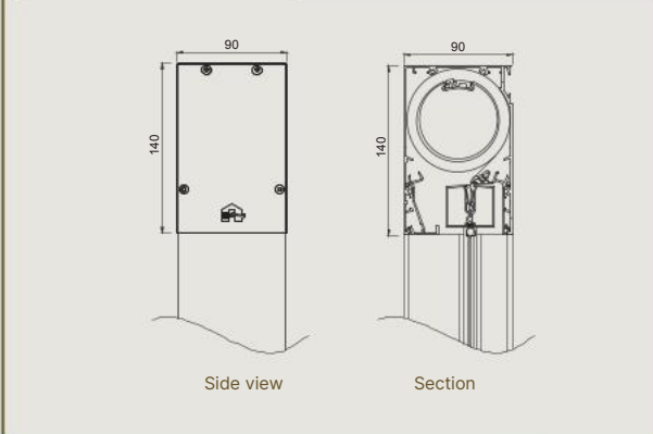
Medium - IM 7A F - head box
