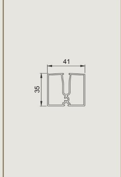
Bottom bar
