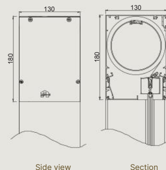
Large - IM 7A - Head box
