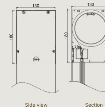
Large - IM 7B - Head box
