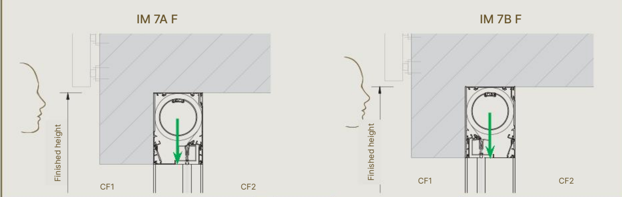
Small - IM 7B F - head box
