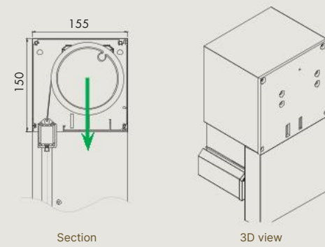
Fixscreen® 150 - IM 7B - Head box
