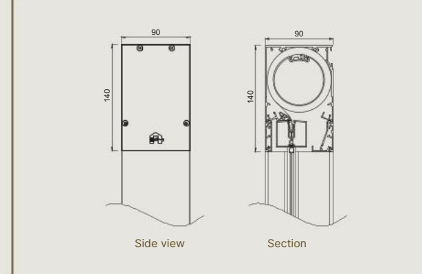
Medium - IM 7B F - head box
