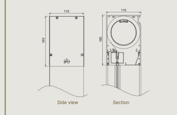
Large - IM 7B F - head box
