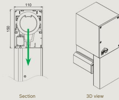
Fixscreen® 100 Slim - IM 7B - Head box
