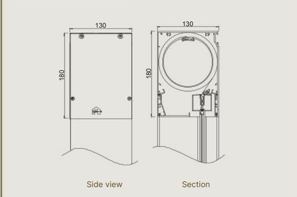
Large - IM 7A F - head box
