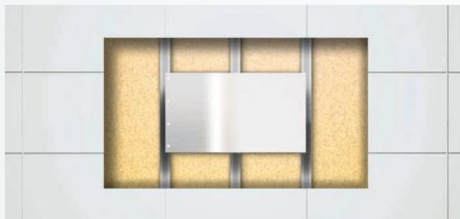
Standard Installationsaufbau hinterlüftete Fassade
