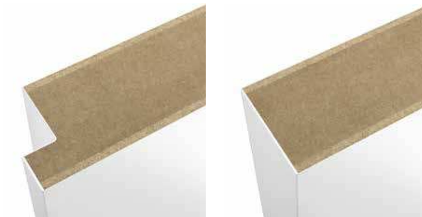
Falcolt kivitel sarkos éllel
