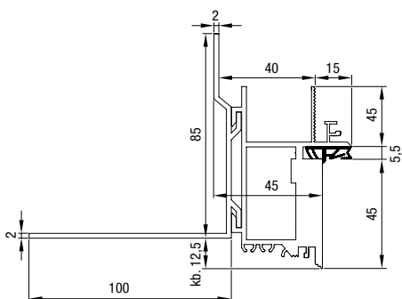
Zeroline tok méretezése
