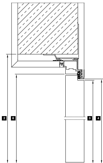
Ellenkezőleg nyíló ajtólap függőleges metszete
