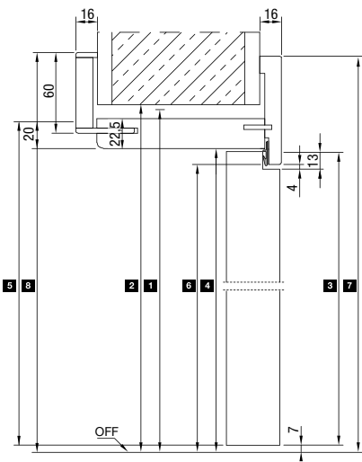
Függőleges metszet
