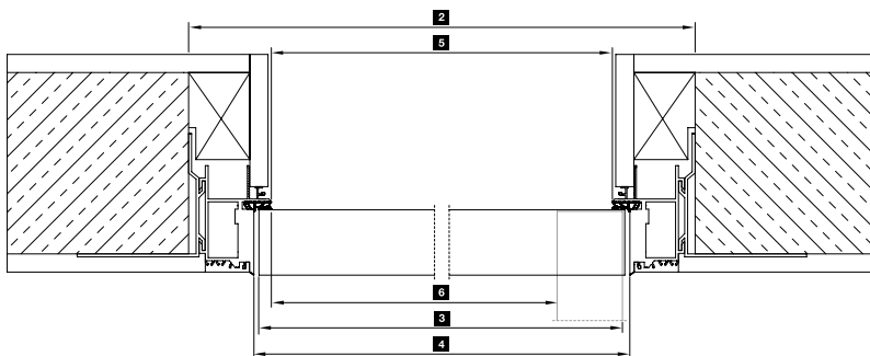
Falcolatlan ajtólap vízszintes metszete
