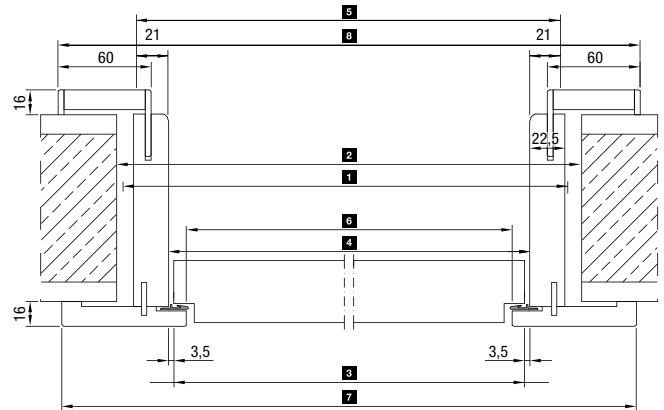
Vízszintes metszetek
