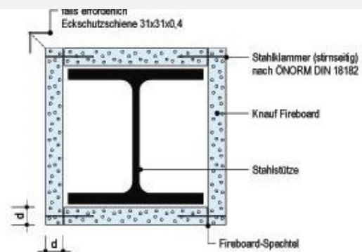
K253-H3 Horizontalschnitt - Einlagig beplankt
